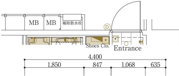
[ B3RTYPE部分図 ]
